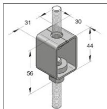
Napinacz zawiesia
